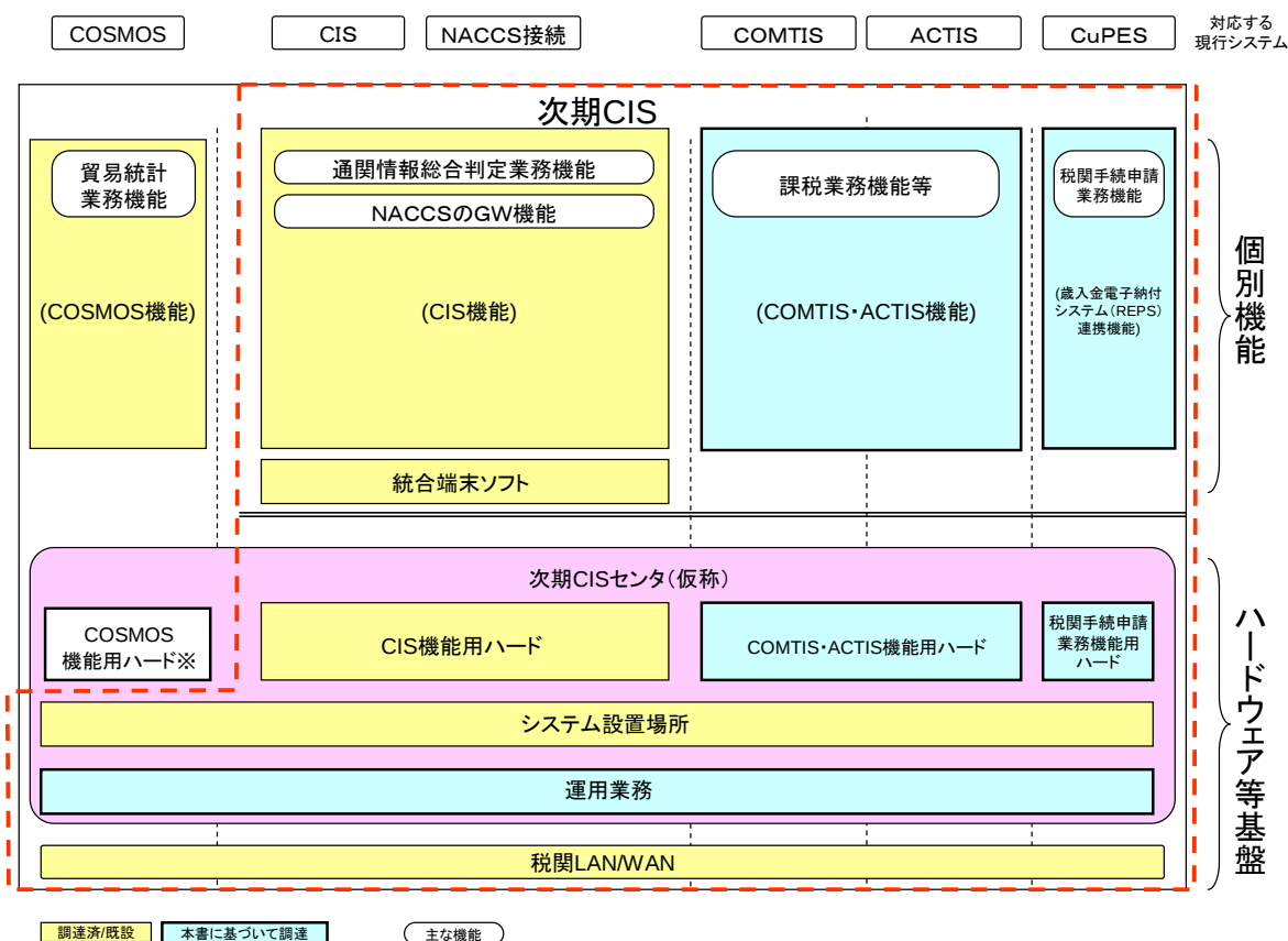
図 2-1 次期 CIS の全体構成（点線で囲った部分が本書で対象とするシステム）
