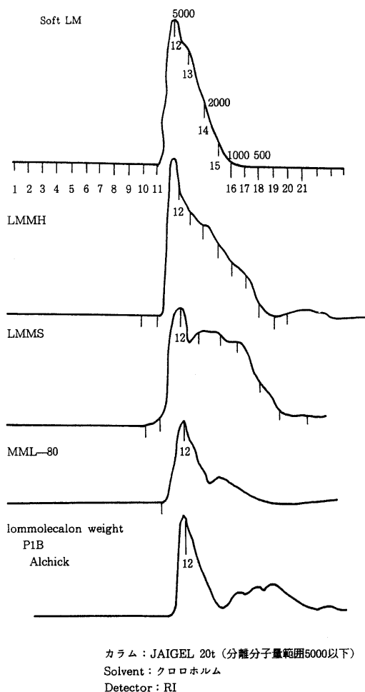
Fig.2 GPC curve of polyisobutylene カラム: JAIGEL 2H(分離分子量範囲 5000 以下) Solvent: クロロホルム Detector: RI
