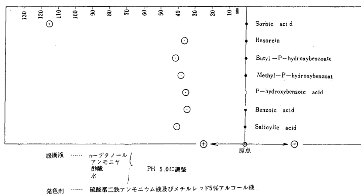
〔Fig.7〕 添加剤電気泳動図 30V/cm 3hrs
