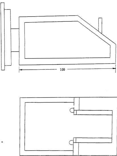
Fig 1 K - 3 試料室
