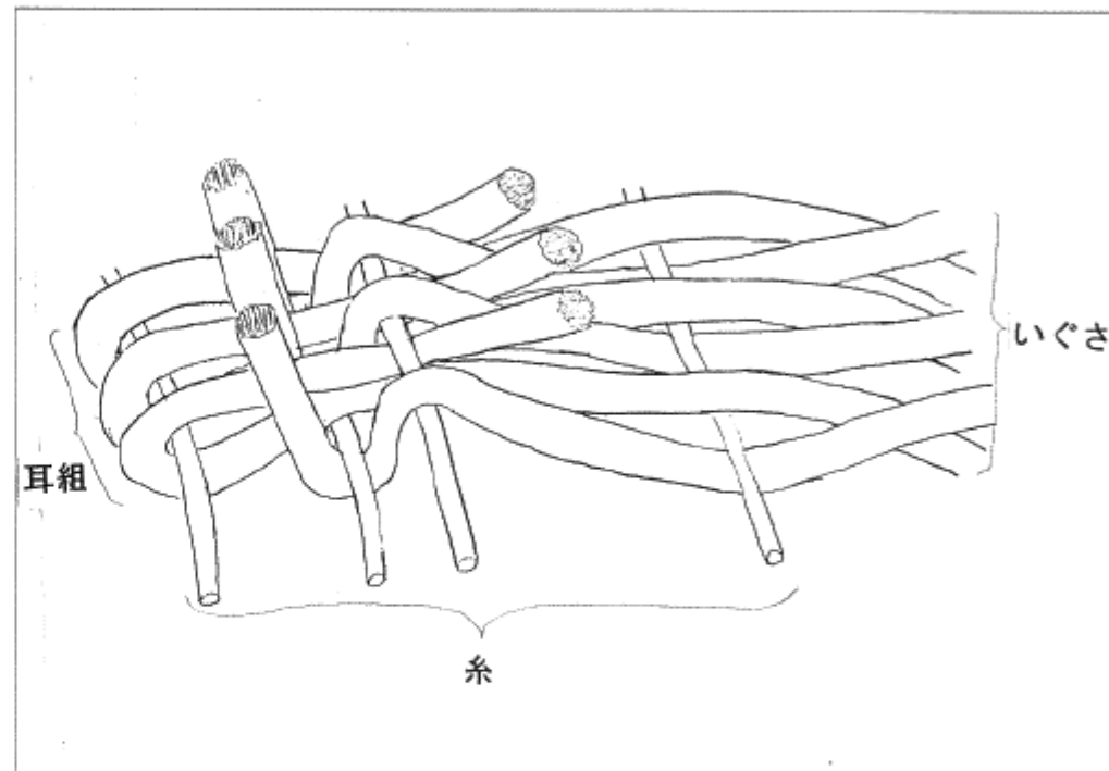
耳毛を製織部分に折り込んだ縁加工（耳組）の拡大図
