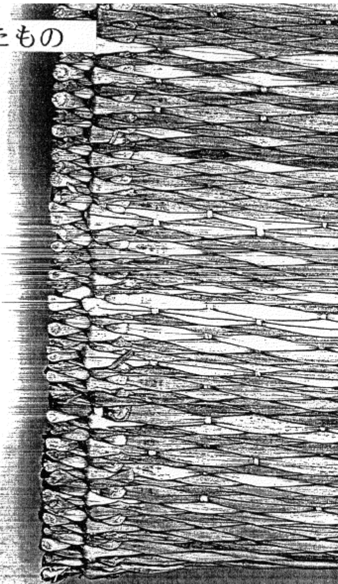
耳毛を製織部分に折り込んだ縁加工（耳組）の拡大図
